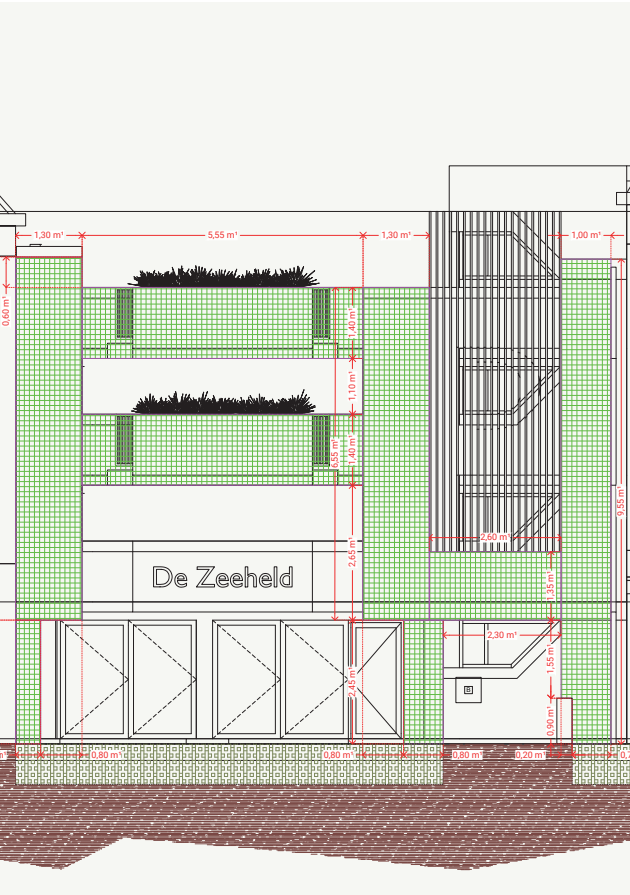
SCHETSTEKENING VAN DE GROENE GEVEL IN WORDING
